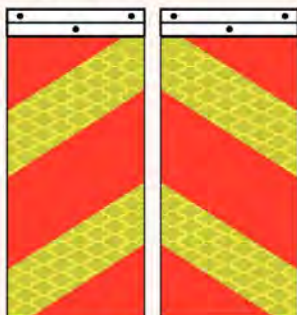
Afmetingen / Dimensions : 283x197mm Aluminium 1mm-Vlak / Plat 2444.04 Geprofileerd / Profile 2425.00
